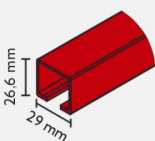
K-075 Nr/No 1 szyna aluminiowa przewodzenia górnego single aluminum rail for upper guidance
