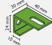
SK-075 Nr/No 1130 kątownik do ścian angle for a wall
