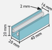
AOG Nr/No 1101 ÷ 1103 przewodnik dolny do szkła 8/10/12 mm lower guidance aluminum rail for glass
